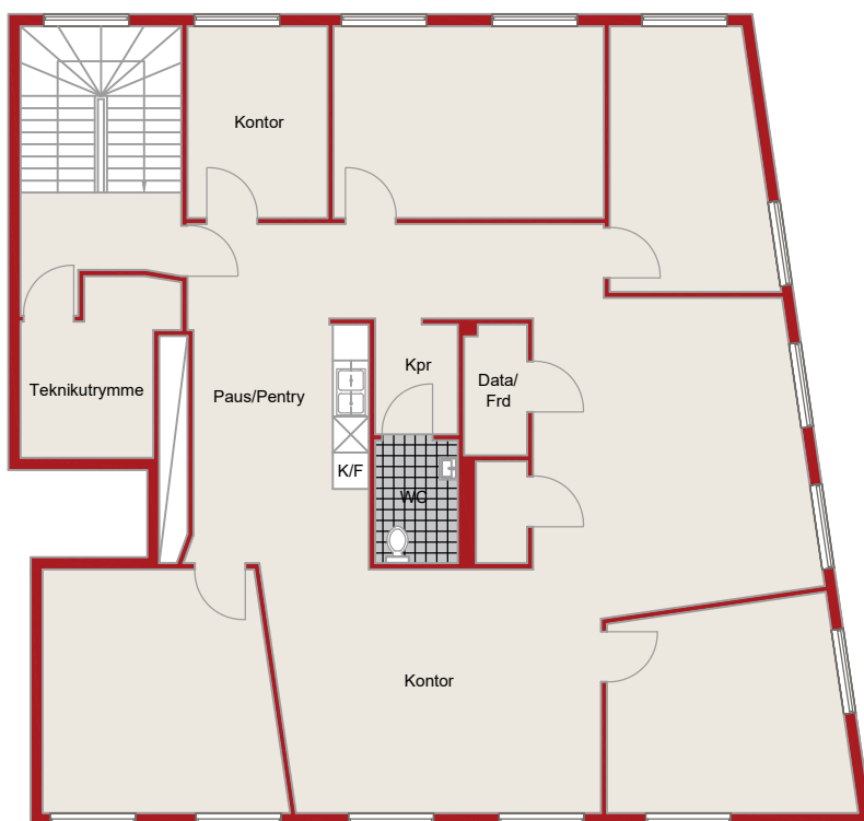
Våning 2
