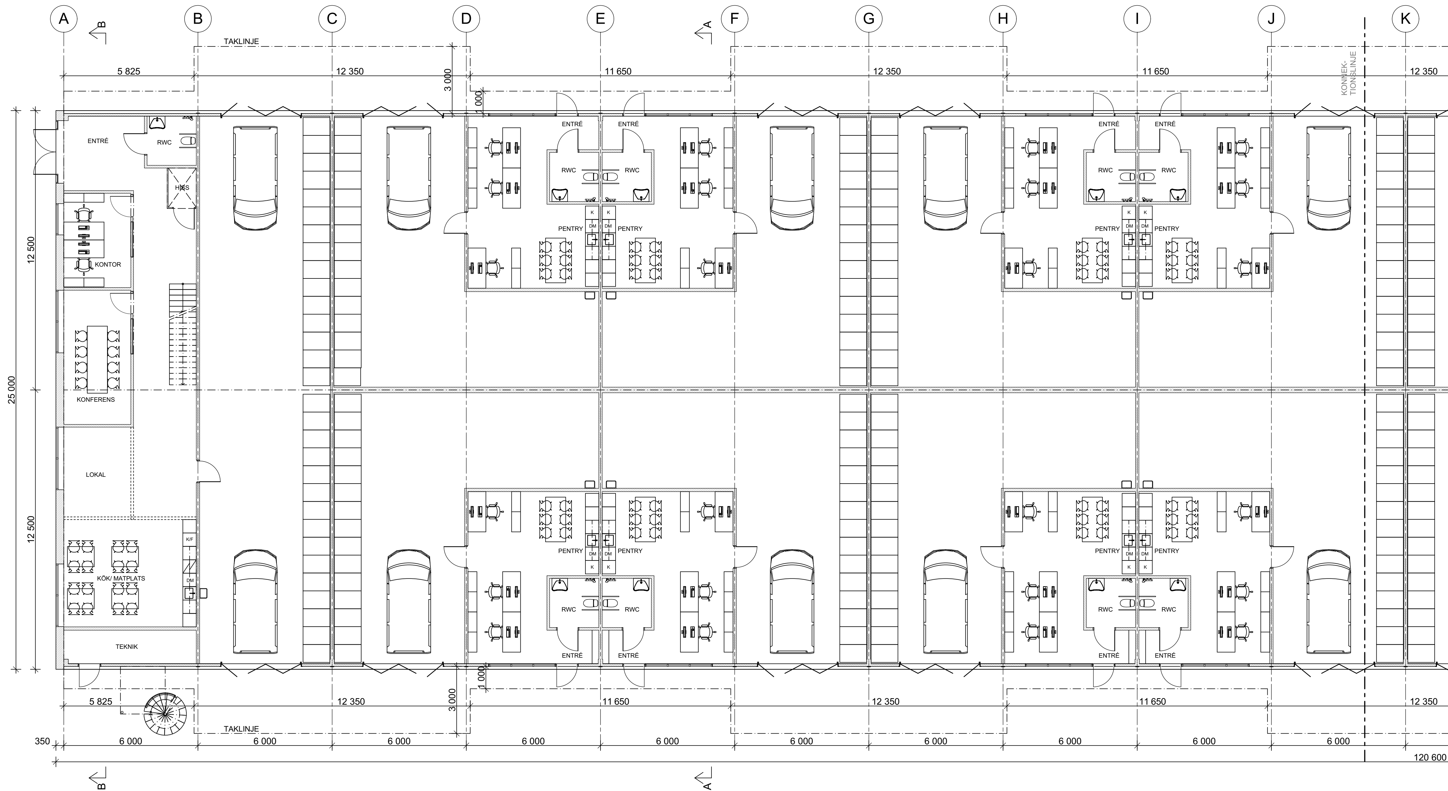
BOTTENPLAN 1:100
