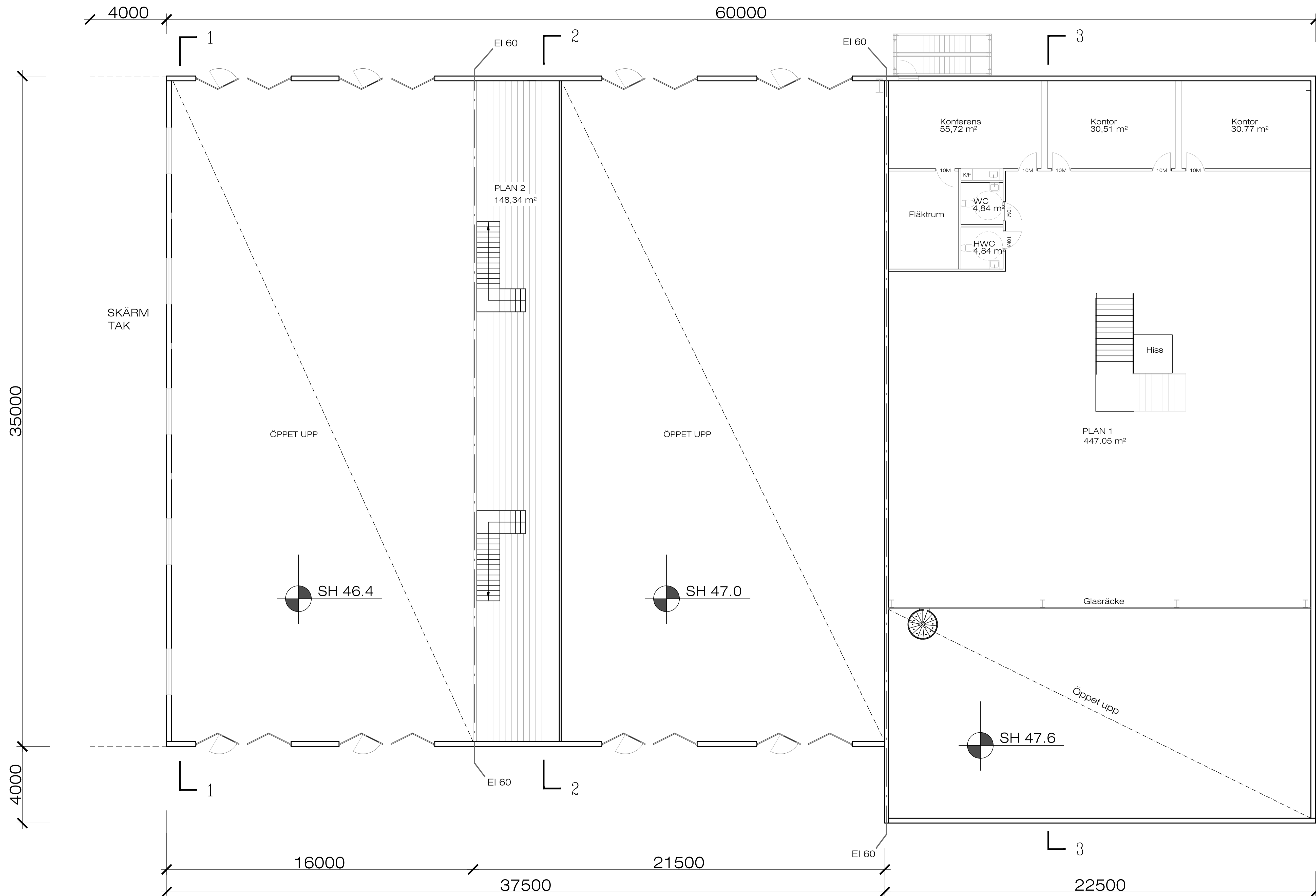
ÖVRE PLAN SKALA 1:100
